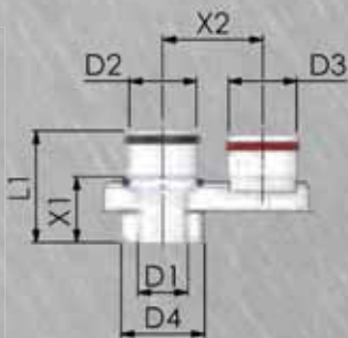
Adapter koncentrično-paralelno
