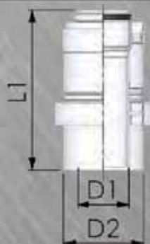
Vodoravni dimovod
