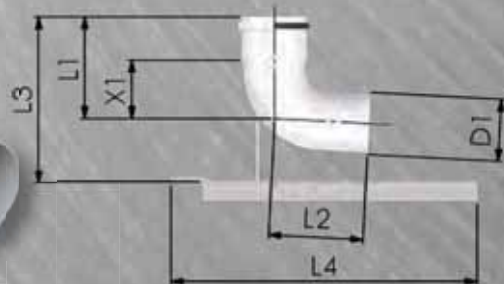
Potporno koljeno
