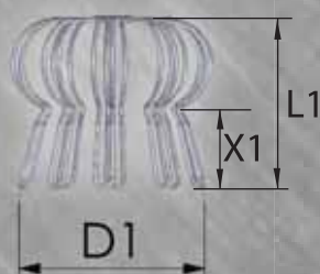
Zaštitna rešetka
