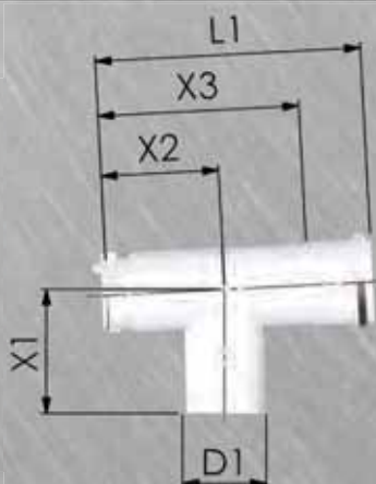
T-komad s revizijom
